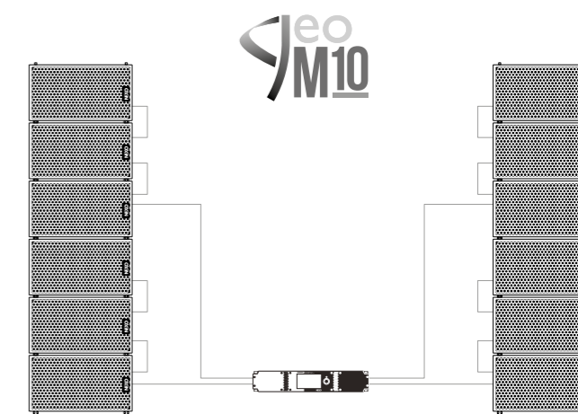
NXAMP4X2 Mk2 alimentant 6 x GEO M10 par cote
