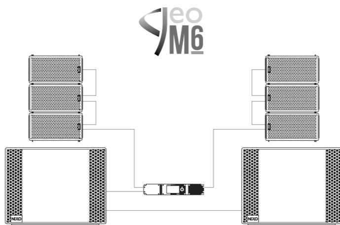
NXAMP4X1 Mk2 alimentant 3 x GEO M6 par cote et 2 x LS18 en mode mono bridgé
