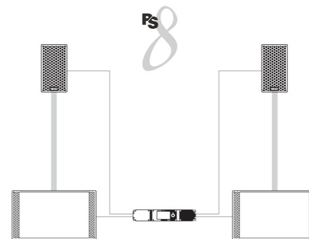
NXAMP4X1 Mk2 alimentant 1 x PS8 et 1 x LS400 Sub par cote
