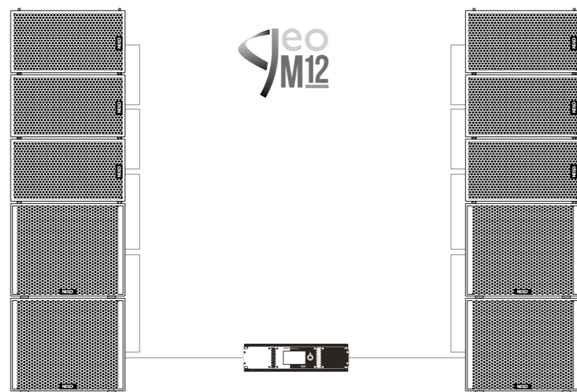
NXAMP4X4 MK2 3 x GEO M12 et 2 x MSUB18 par cote
