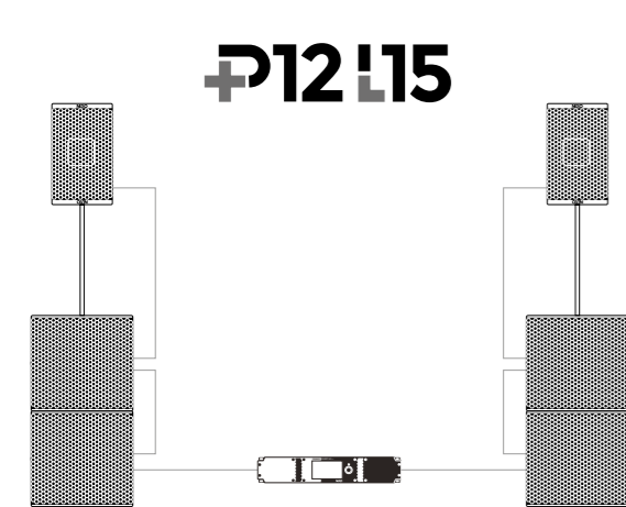
NXAMP4X2 Mk2 alimentant 1 x P12 et 2 x L15 par cote
