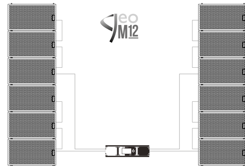
NXAMP4X4 MK2 alimentant 6 x GEO M12 par cote
