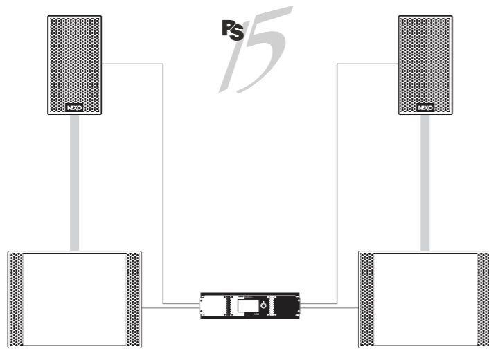
NXAMP4X4 MK2 alimentant 2 x PS15 et 2 x LS18 par cote
