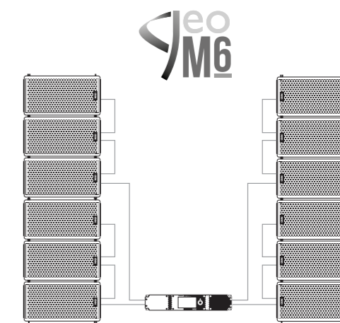
NXAMP4X1 Mk2 alimentant 6 x GEO M6 par cote
