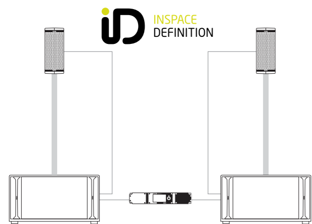
NXAMP4X1 Mk2 alimentant 1 x ID24 et 1 x IDS110 Sub par cote
