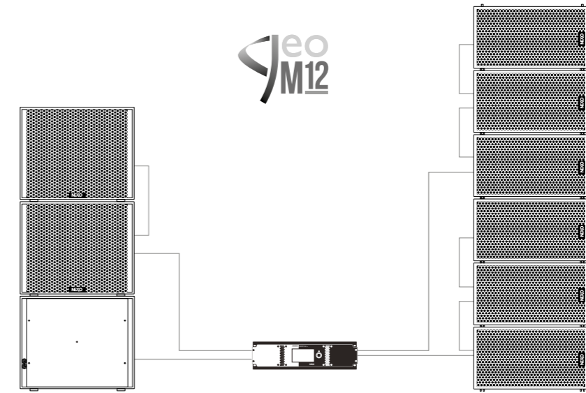
NXAMP4X4 MK2 alimentant 3 x MSUB18 (dont un en mode cardio) et 6 x GEO M12
